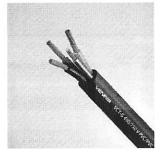
ตัวอย่างตู้โหลดเซ็นเตอร์ สำหรับเบรกเกอร์ 3 เฟส ตัวอย่างหางปลา (Ring Terminal) ตัวอย่างสายจนวนหุ้ม 2 ชั้น (VCT)
