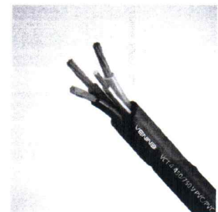
ตัวอย่างสายฉนวนหุ้ม 2 ชั้น (VCT)
